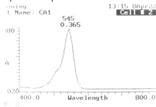
Gambar I. Panjang Gelombang Maksimum Rhodamin B
