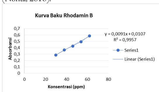
Gambar 2. Persamaan linier & kurva baku Rhodamin B
