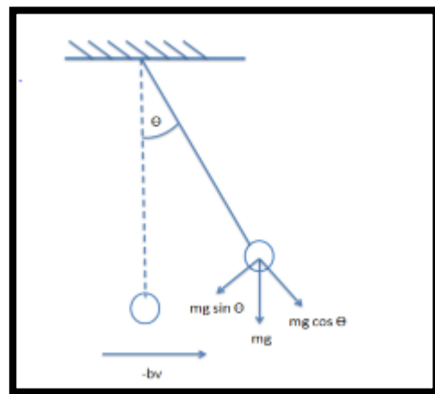
Gambar 1. Bandul Sederhana
