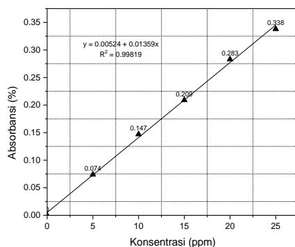
Gambar 3. Gambar Kurva Hubungan Absorbansi terhadap Konsentrasi
