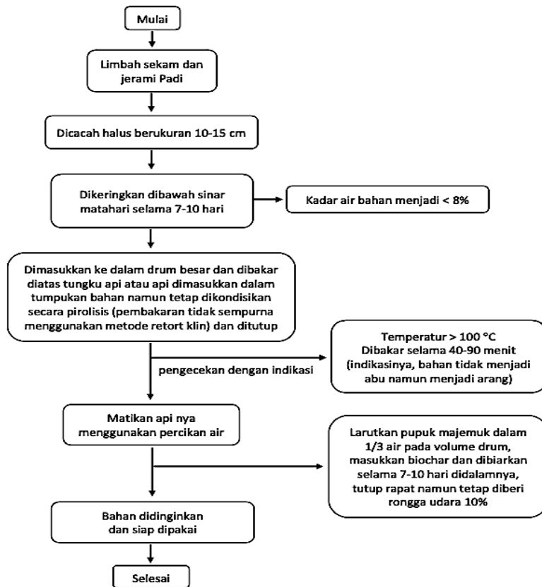
Gambar 1. Metode Pembuatan Biochar
